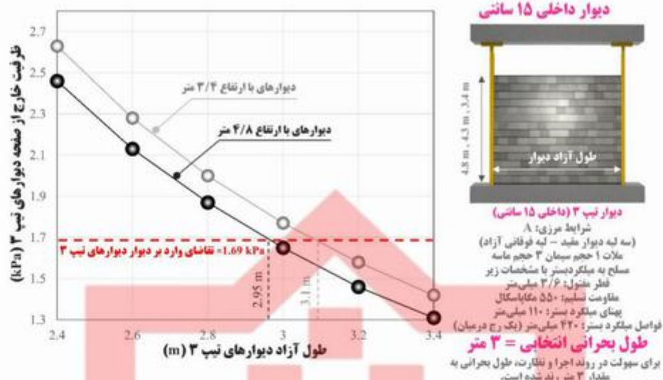
شکل پ-۵-۸ تعیین طول بحرانی برای دیوارهای تیپ ۳ (دیوارهای داخلی ۱۵ سانتی)
