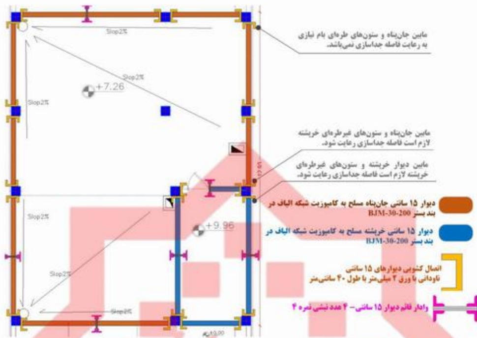
شکل پ-۱۰- تیپ‌بندی دیوارها، جانمایی وادارهای قائم و اتصالات کشویی در بام و خریشته
